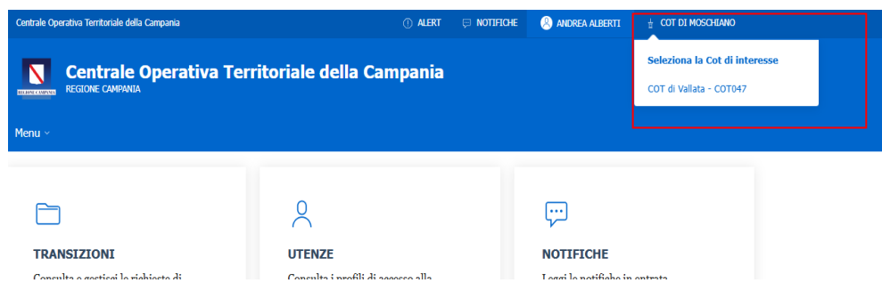
Figura 47 - Selezione COT
