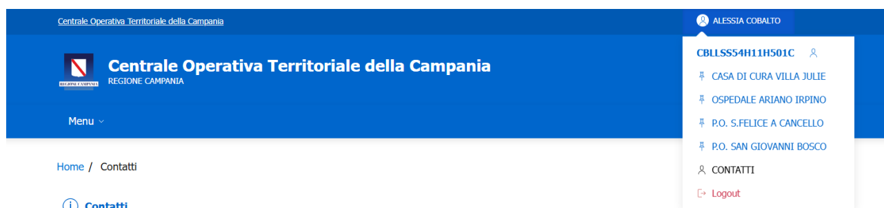
Figura 49 - Sezione Contatti
